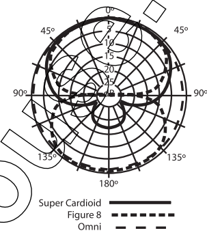
C03U POLAR PATTERN
