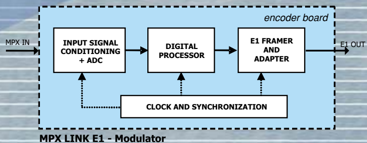
MPX LINK E1 - Modulator
